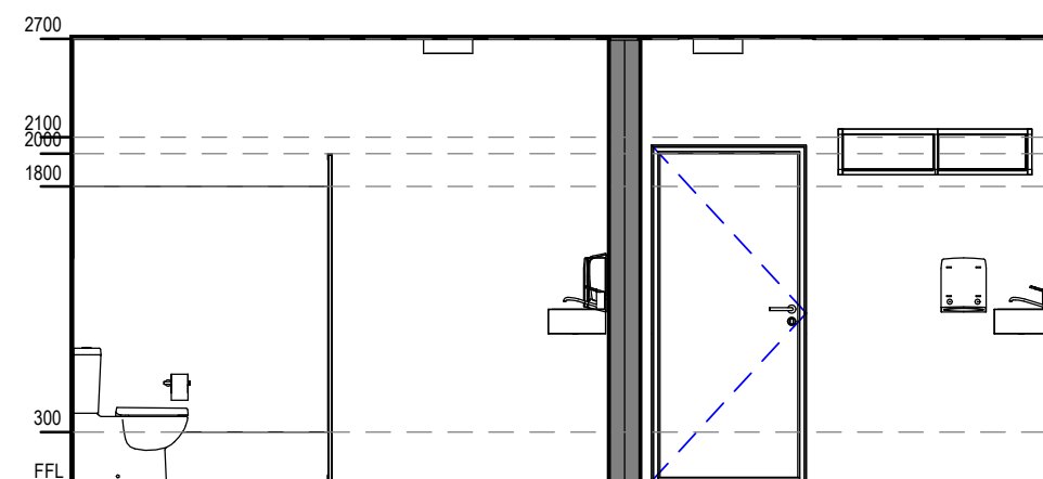
11 MALE STAFF & MALE ST WC ELE 11 SCALE: 1 : 50
