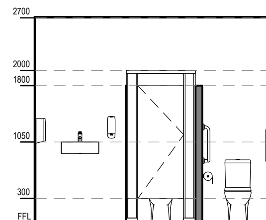
12 MALE STAFF WC ELE 12 SCALE: 1 : 50
