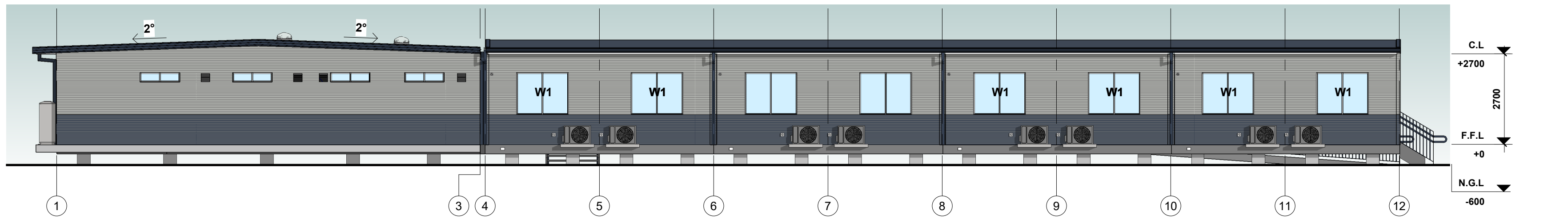
1 REAR ELEVATION SCALE: 1 : 100
