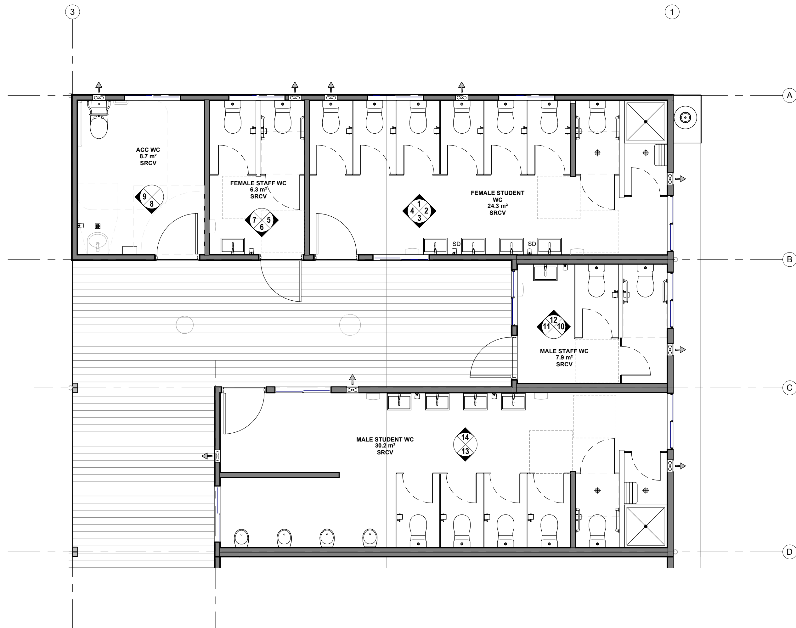
1 TOILET FLOOR PLAN SCALE: 1 : 50
