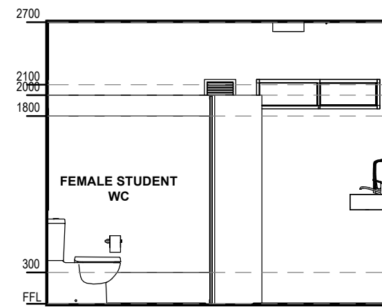
2 FEMALE ST WC - ELE 2 SCALE: 1 : 50
