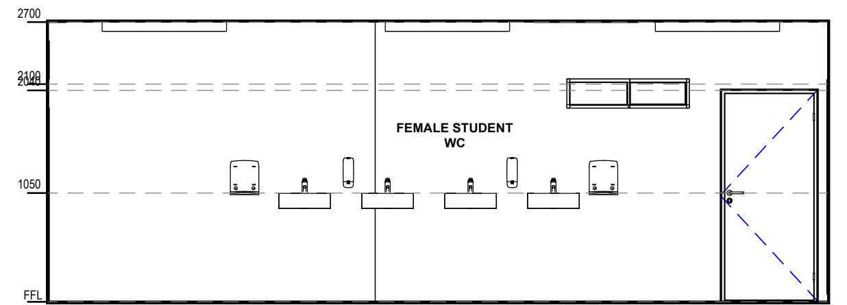
3 FEMALE ST WC - ELE 3 SCALE: 1 : 50
