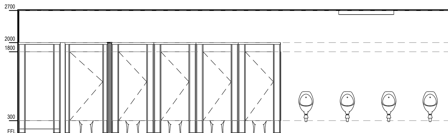
13 MALE STUDENT WC ELE 13 SCALE: 1 : 50
