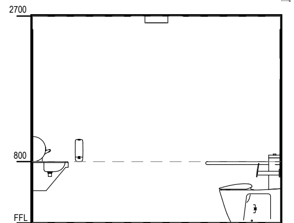
9 ACC WC ELE 9 SCALE: 1 : 50
