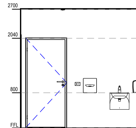
8 ACC WC ELE 8 SCALE: 1 : 50
