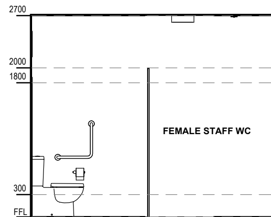
5 FEMALE STAFF WC - ELE 5 SCALE: 1 : 50
