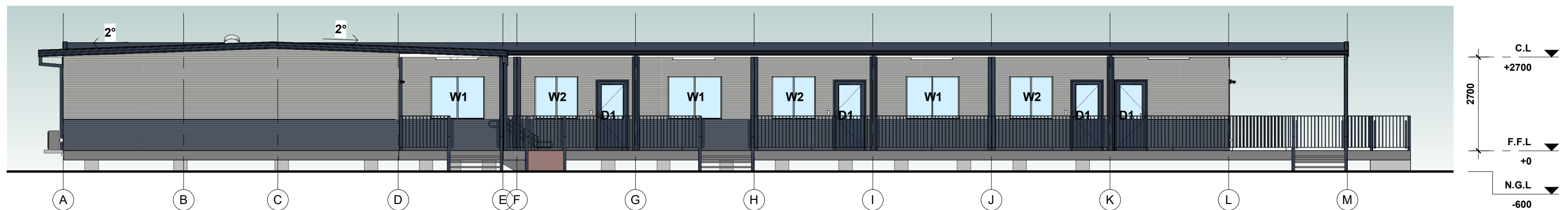
4 LEFT SIDE ELEVATION SCALE: 1 : 100
