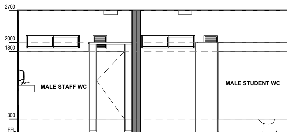
10 MALE STAFF & MALE ST WC ELE 10 SCALE: 1 : 50
